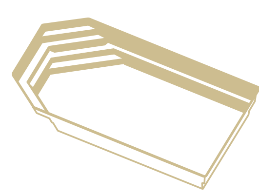
Tanzanite 8' Longueur : 8 m Largeur : 4,06 m Profondeur : 1,46 m
