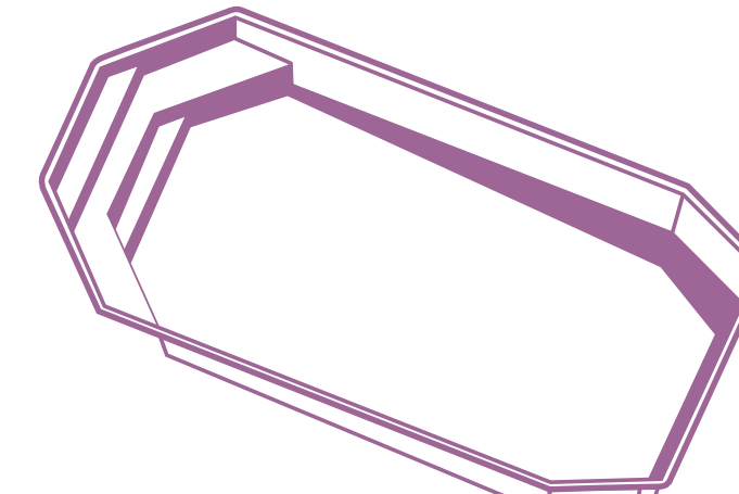
Cristal Longueur : 7 m Largeur : 3,50 m Profondeur : 0,93 - 1,53 m
